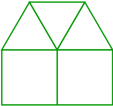
Vertex: 3.3.3.4.4
