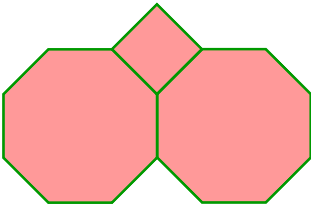
Vertex: 4.8.8
